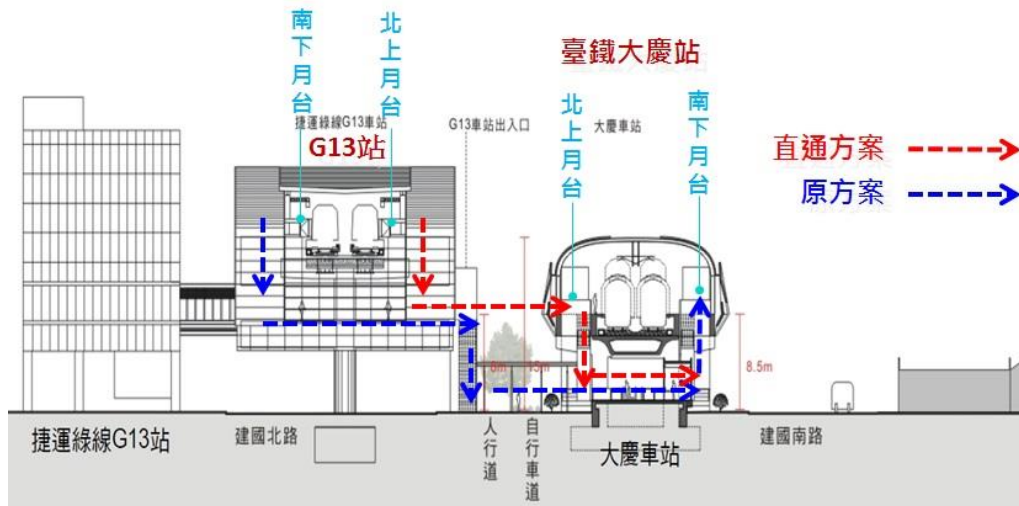
圖 15 原方案與直通方案轉乘動線圖
