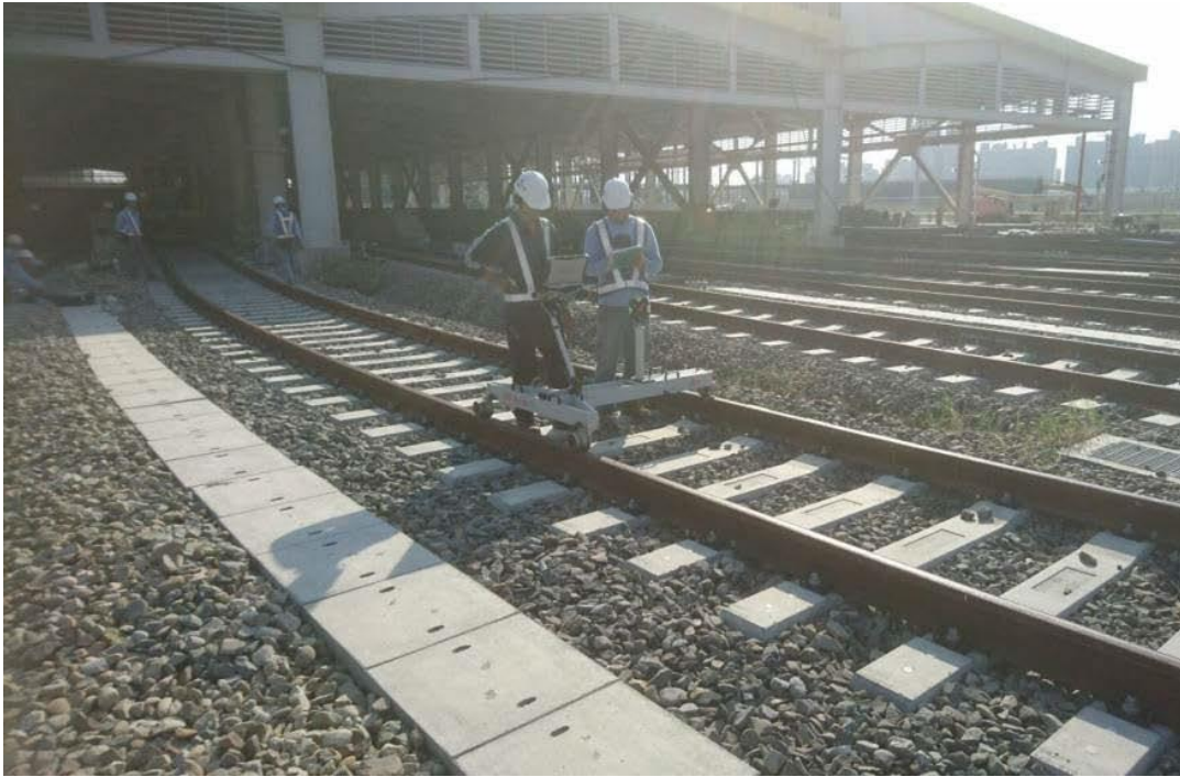
圖 7 北屯機場軌道施作現況
