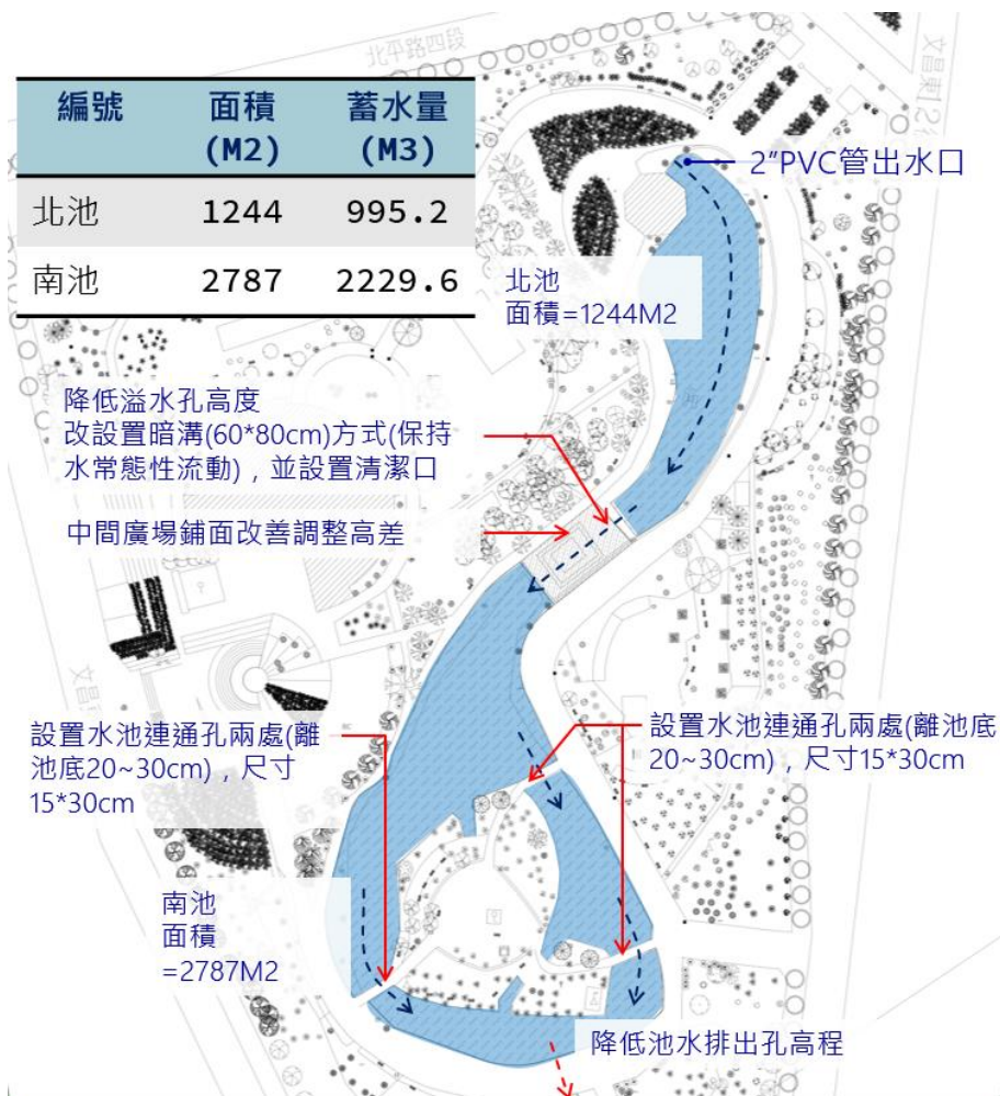
北屯兒童公園水池現況排水圖
