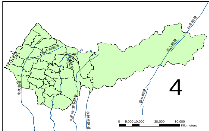
大臺中地區斷層
