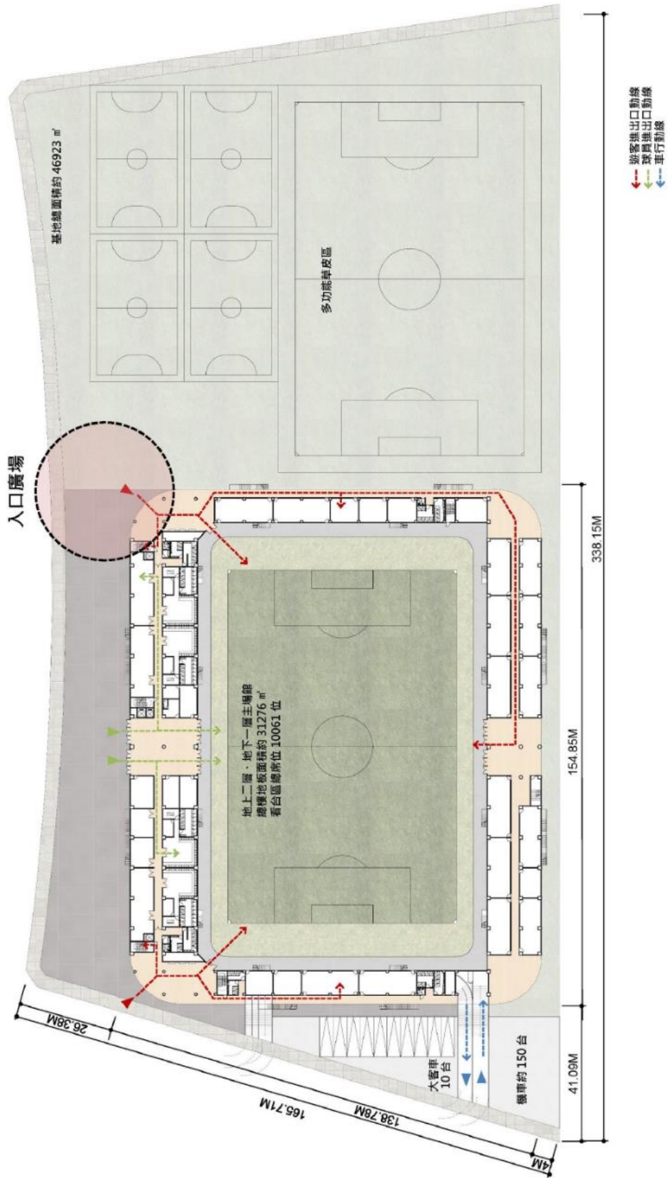
圖 2 足球場配置示意圖
