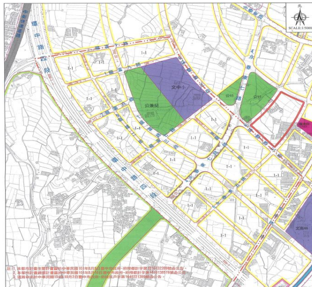
圖 1 臺中市都市計畫(整體開發地區單元五)細部計畫圖
