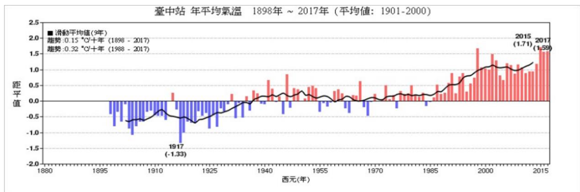
圖1 臺中市百年溫度變化
